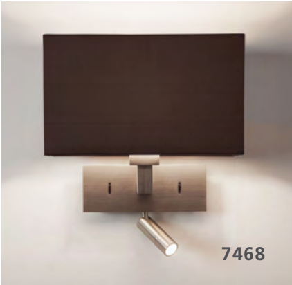
PARK LANE AP LED αηλικά / wallfitting E14 40W & LED 1W βάση: ματ νίκελ, χρώμιο, μπρονζέ base: matt nickel, chrome, bronze H20,5cm x L25cm x Ø13,5cm extra καπέλλο: λευκό, μαύρο, μπεζ, γκρι extra shade: white, black, beige, grey
