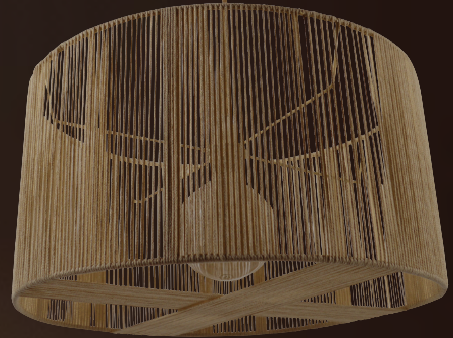
DIANA 50 / PATO κρεμαστό / pendant E27 60W Ø50 x H27cm περαστό με πάτο λινάτσα with burlap bottom σχοινί καλώδιο / rope cable
